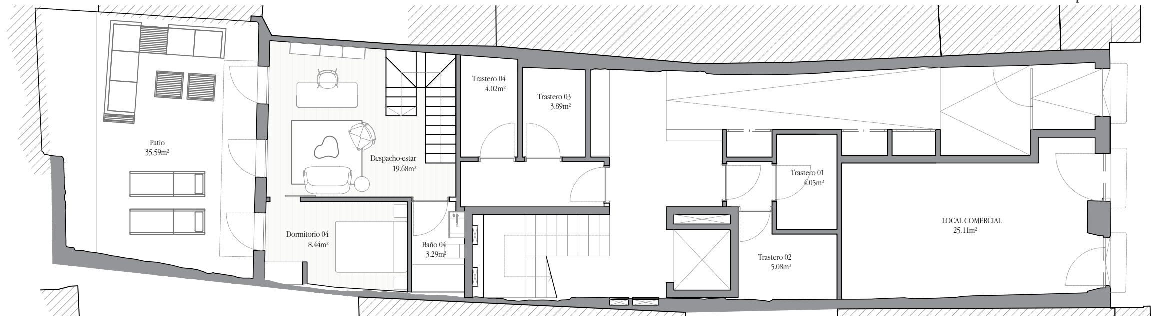
Planta baja
